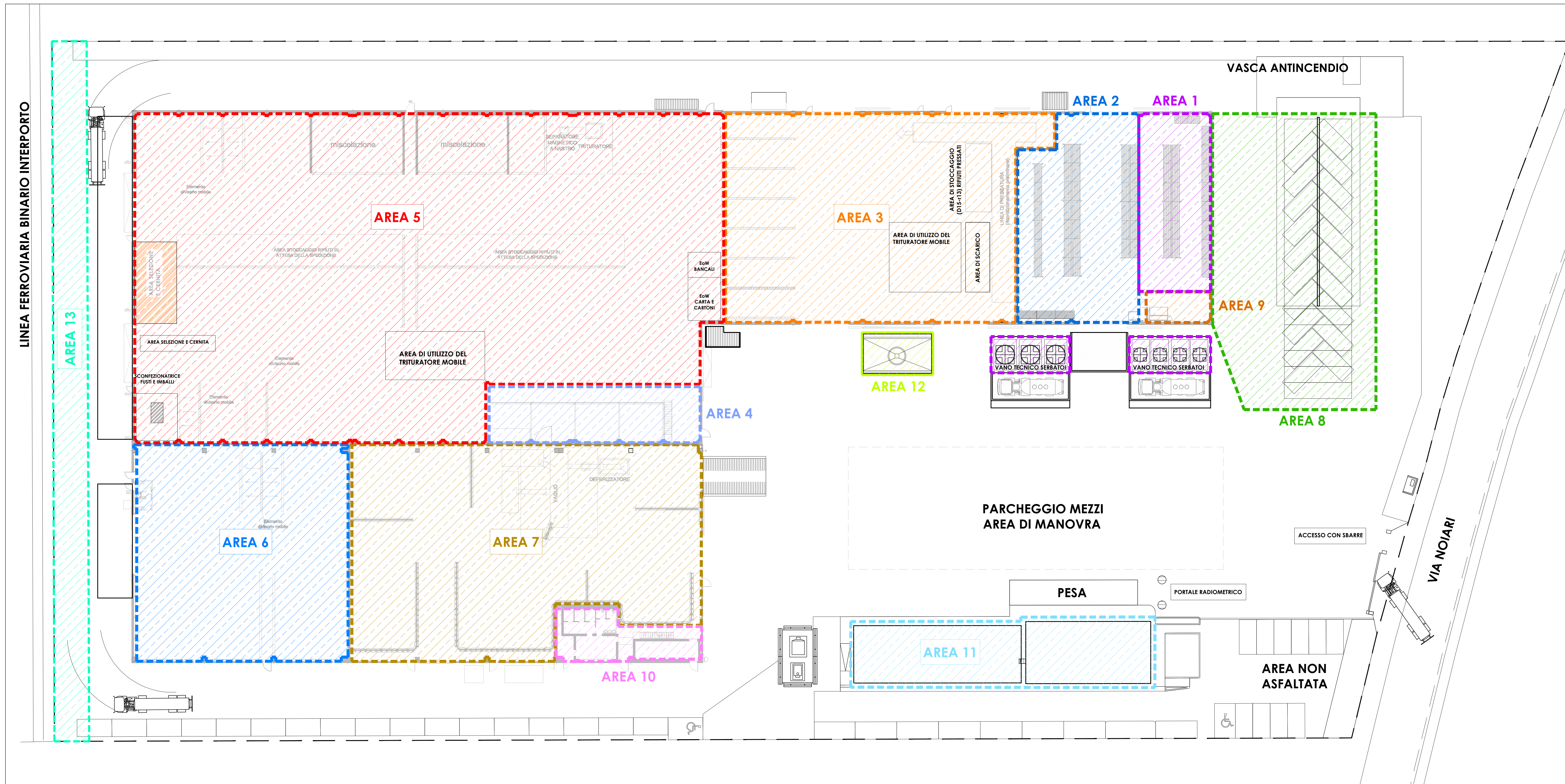
PLANIMETRIE LAYOUT MACROAREE DI STOCCAGGIO scala 1:250
